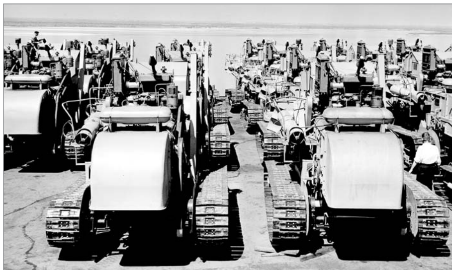
Комбайны «СКГ-3» Хабаровского завода «Дальдизель» перед отправкой на Кубу. Хабаровск, июнь 1962 г. Фотограф Н. Суровцев. РГАКФД. Арх. № 1-59363.
